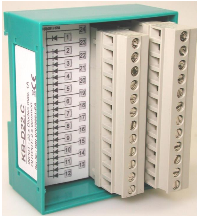
KB-D22.C Klemme 1-12 13-24
